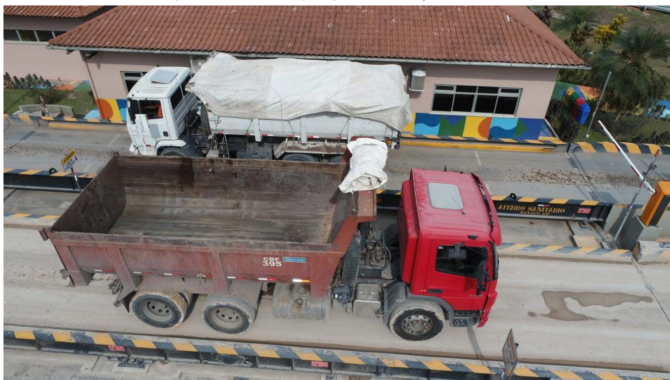
Figura 36: Processo de pesagens nas balanças de entrada e Saída
