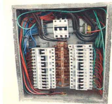
Quadro de distribuição do pavilhão Virgínia Amorim.
